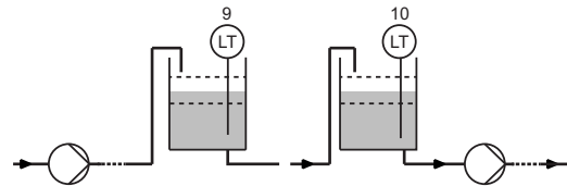
Рис. 134 Обзор мест расположения датчика
