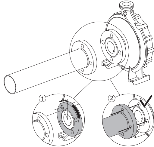
Рис. 93 Свободный фланец
