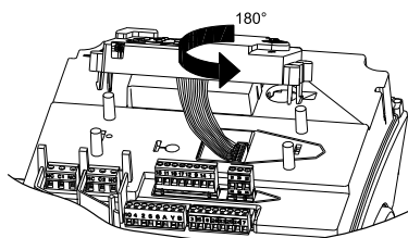
Рис. 71 Поворот пластмассовой крышки
