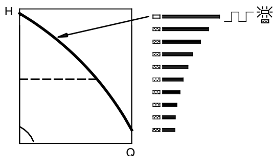
Рис. 19 Эксплуатация при максимальной характеристике
