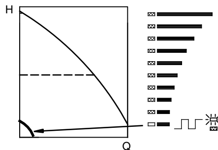
Рис. 18 Эксплуатация при минимальной характеристике
