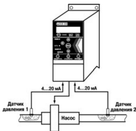
Рисунок 4.6 - Схема установки
